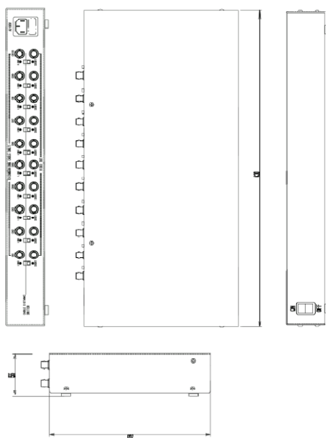
■寸法図(単位: mm)
