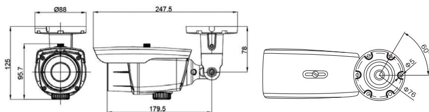
寸法図 (mm)
